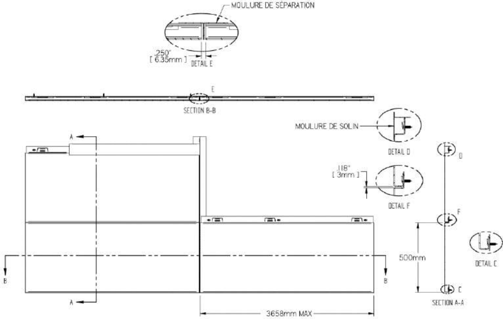
▲ Vue en élévation, coupe et plan des panneaux
